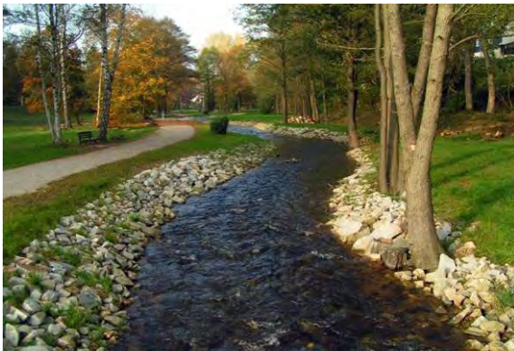
eingeschränkte Querprofilusbildung
