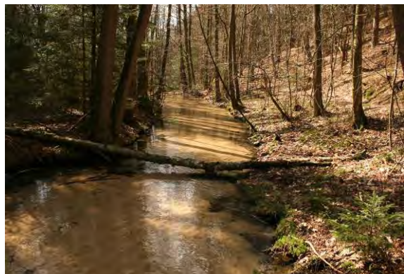
Sohlenkerbtal
