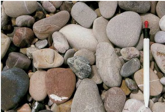
Schotter
