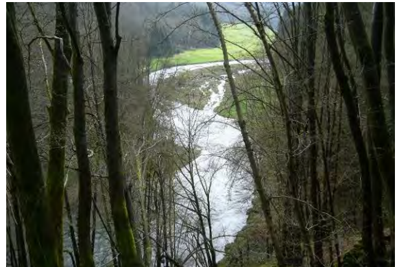
Nebengerinne
