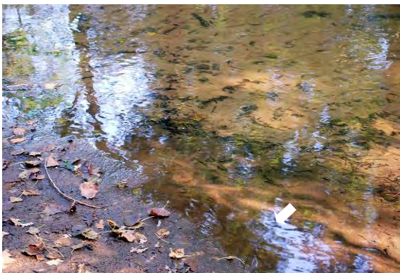
Feindetritus
