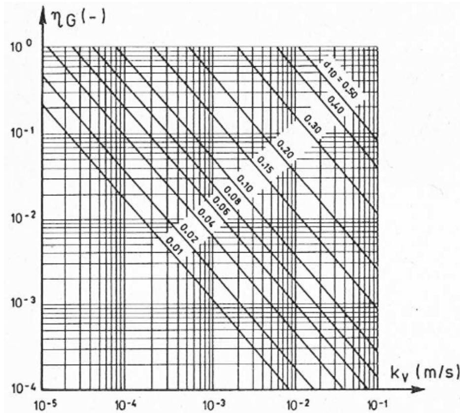
Abbildung 31 Bestimmungsdiagramm für Abminderung \eta_G
