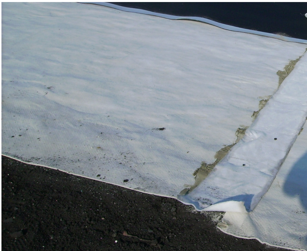
Abbildung 8 geosynthetische Tondichtungsbahn Überlappungszone (Querstoß) mit aufgetragener Bentonitpaste Foto: Naue GmbH & Co. KG
