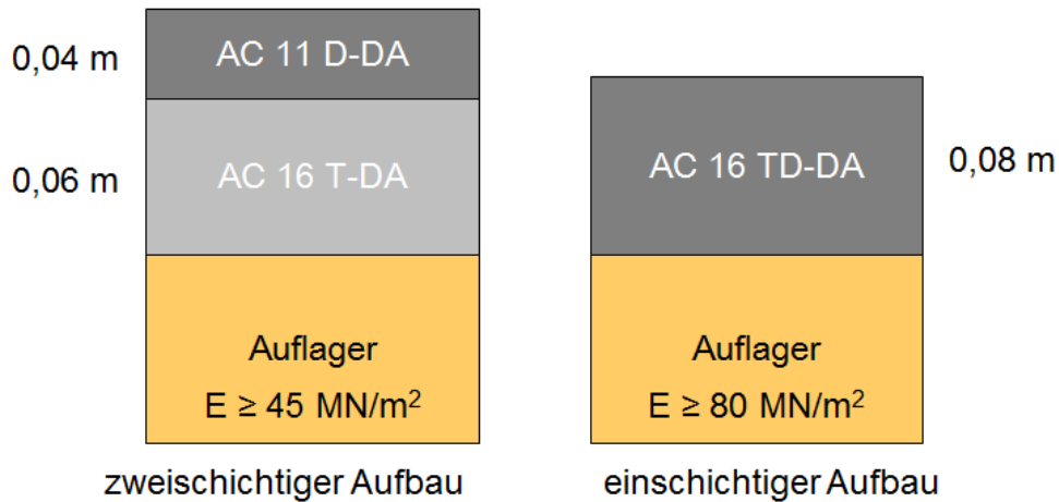
Abbildung 11 alternative Bauweisen für Deponieasphalt
