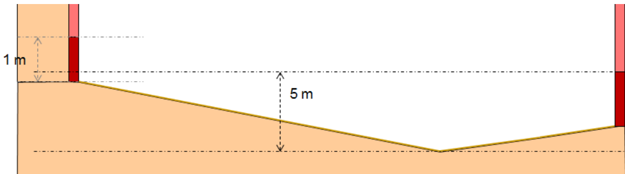
Abbildung 1 Ermittlung der Ausbauhöhe von Dichtwänden nach den Anforderungen an das Basisabdichtungssystem
