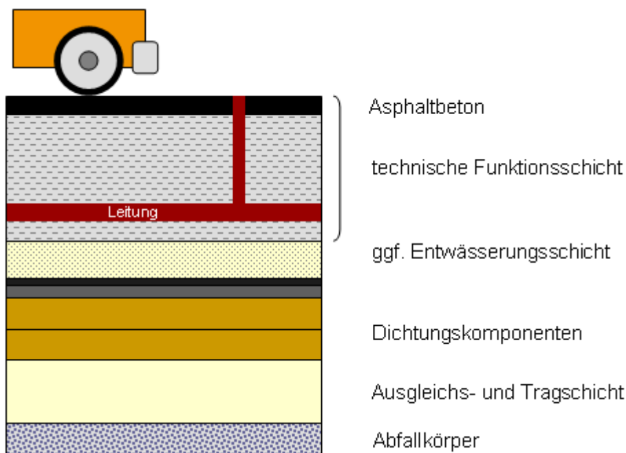
Abbildung 22 Schemadarstellung einer entkoppelten Funktionsschicht
