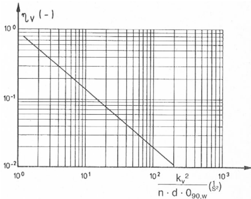
Abbildung 32 Bestimmungsdiagramm für Abminderung \eta_v
