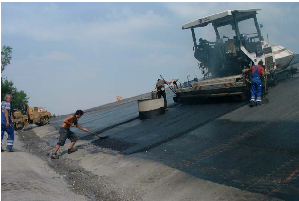
Abbildung 12 Einbau von Deponieasphalt mit einem Fertiger
