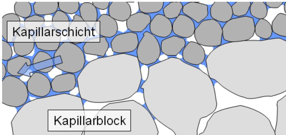
Abbildung 13 Wirkungsprinzip einer Kapillarsperre
