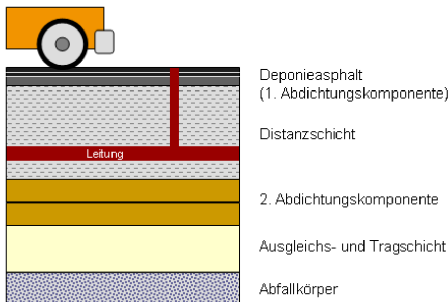
Abbildung 23 Schemadarstellung einer teil-entkoppelten Funktionsschicht
