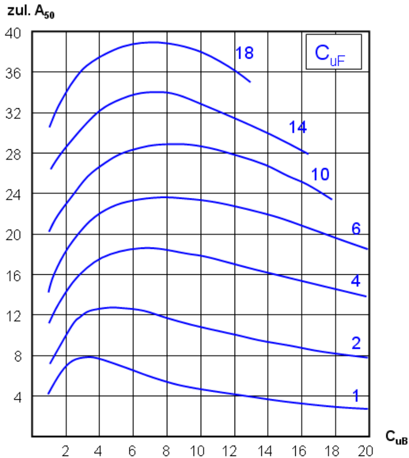
Abbildung 28 Filterdiagramm nach Cistin/Ziems
