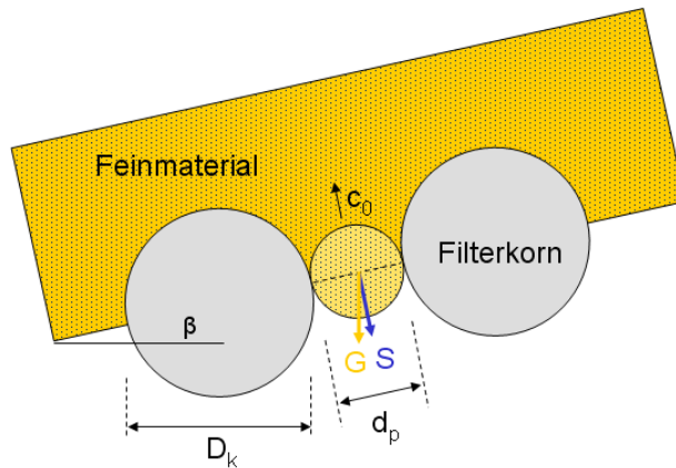
Abbildung 30 Schemadarstellung Kontaktterrosion nach Davidenkoff
