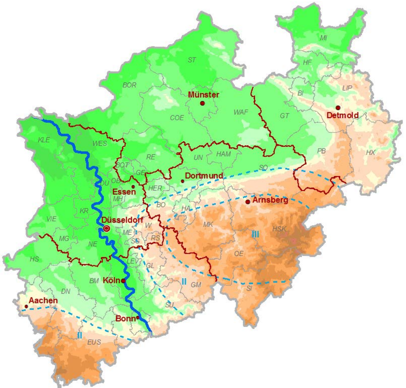
Abbildung 36 Frosttiefezonen in Nordrhein-Westfalen Die Zonen II und III sind hellblau markiert; die restliche Fläche gehört zu Zone I.
