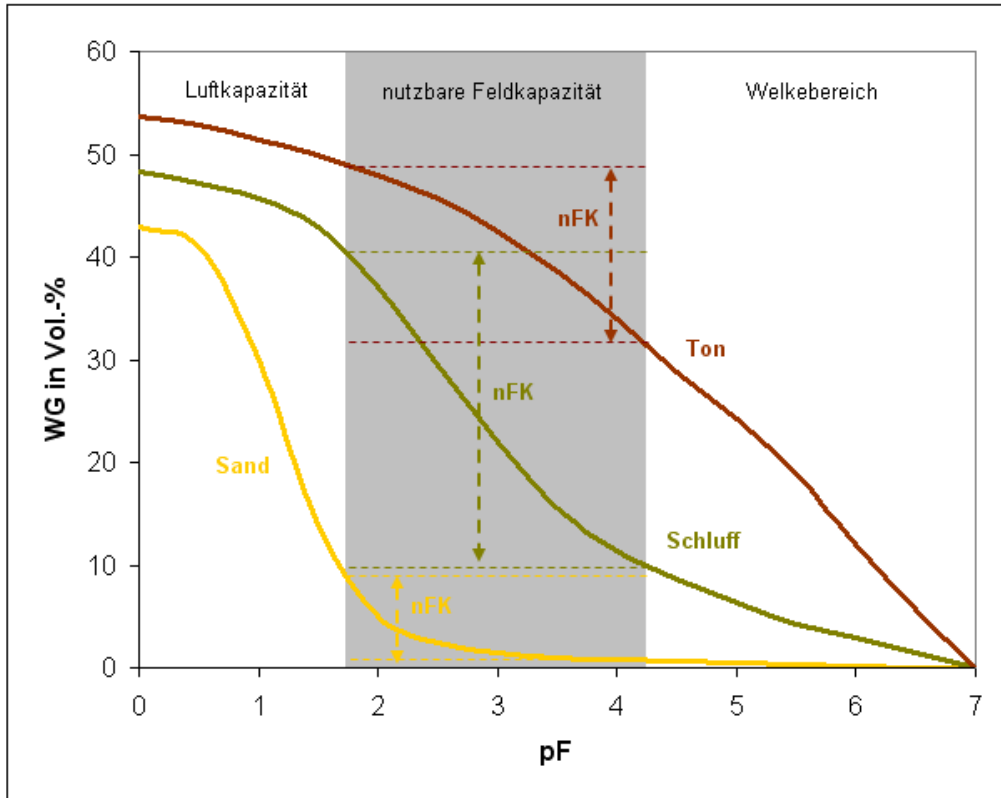
Abbildung 26 pF-Kurve verschiedener Bodenmaterialien
