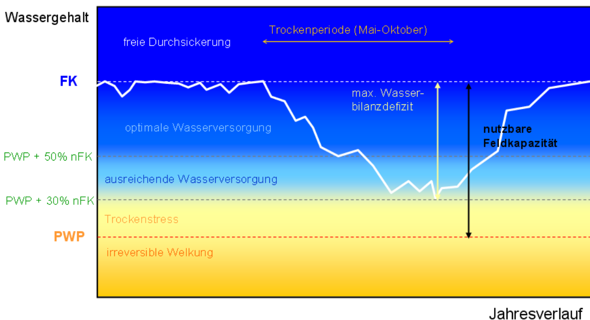
Abbildung 19 Bodenwasservorrat im Jahresverlauf
