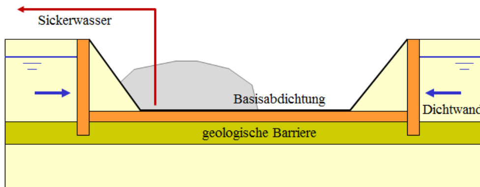
Abbildung 2 Beispiel Grubendeponie ohne freie Entwässerung
