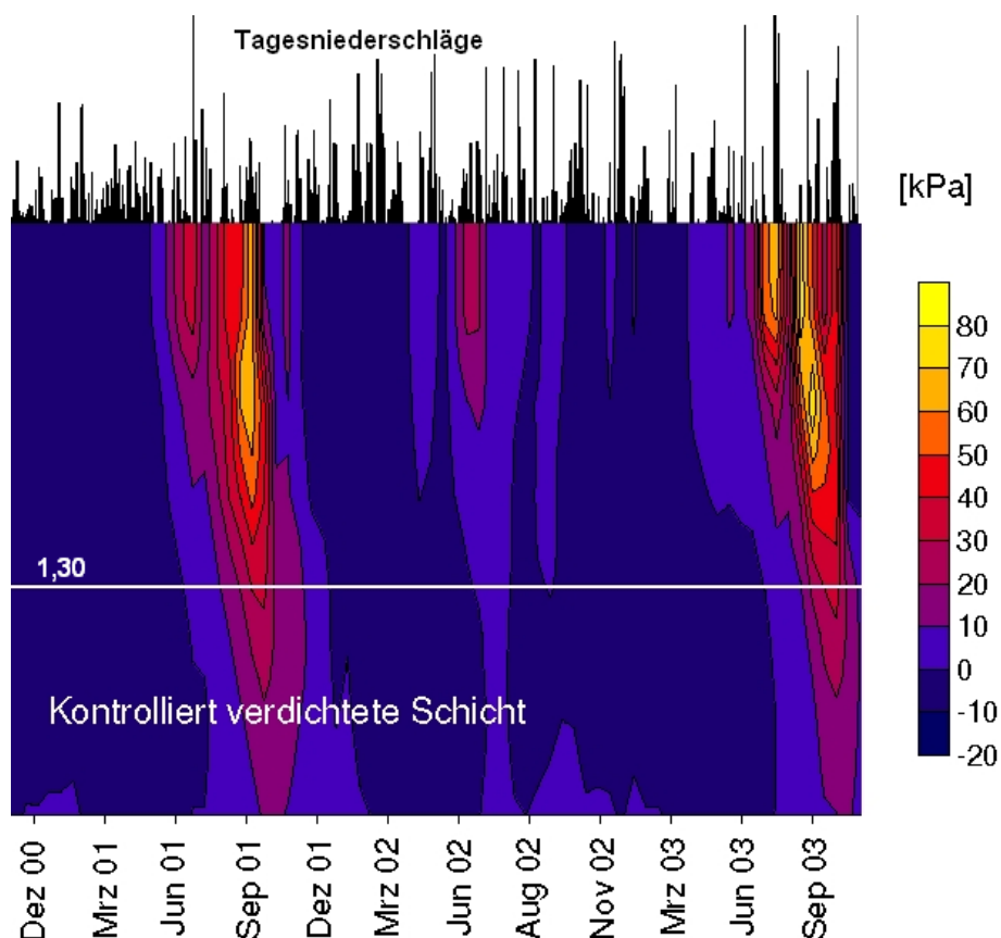
Abbildung 27 Wasserspannung in einer Rekultivierungsschicht Zeitlicher Verlauf in einem Beispiel Quelle: Ruhr-Universität Bochum, Prof. H. Zepp
