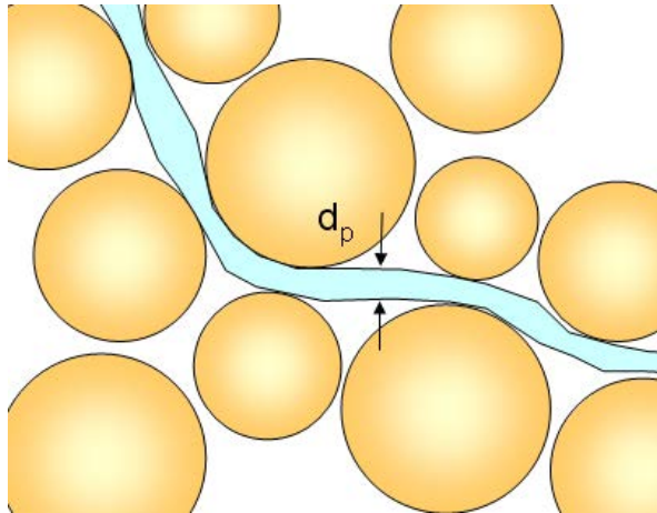
Abbildung 29 Äquivalenter Porenkanaldurchmesser
