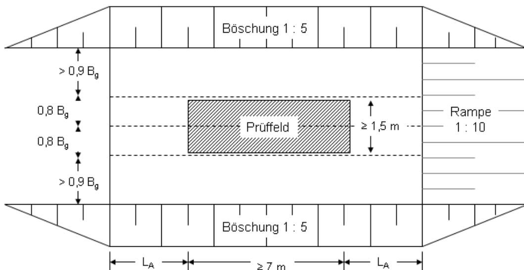
Abbildung 3 Abmessungen für ein Probefeld
