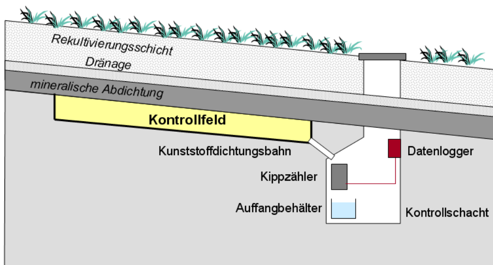
Abbildung 16 Gestaltungsvorschlag für ein Kontrollfeld am Beispiel einer mineralischen Abdichtungsschicht
