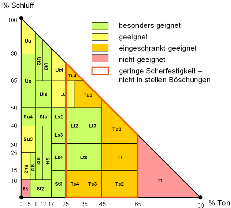
Abbildung 20 Eignung der Feinbodenarten als Rekultivierungsmaterial nach [36] , (Bodendiagramm nach [1])
