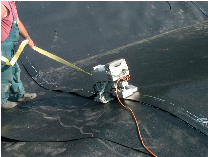
Abbildung 4 Verschweißen zweier Kunststoffdichtungsbahnen
