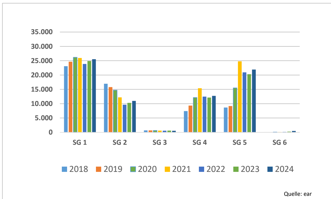
Abbildung 38: Von öffentlich-rechtlichen Entsorgungsträgern in Nordrhein-Westfalen zur Abholung bereitgestellte Mengen an Elektro- und Elektronikgeräten 2018 bis 2024 nach Sammelgruppen gemäß § 14 Abs. 1 ElektroG
