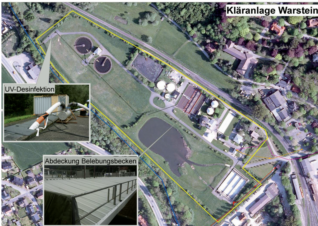
Kläranlage Warstein
