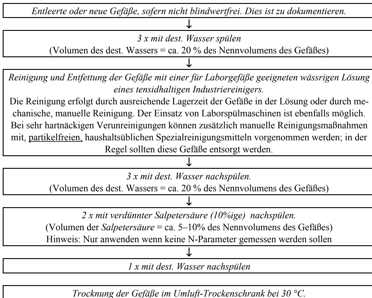
Abbildung 3.2: Ablaufschema zur Reinigung von Probengefäßen aus Kunststoff, bevorzugt für die Bestimmung anorganischer Parameter
