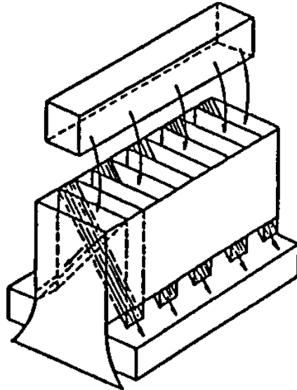
Abbildung 5.5: Riffelteiler
