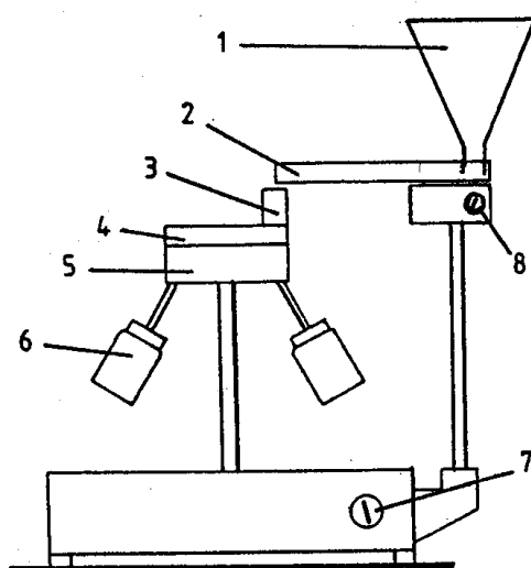
Abbildung 5.6: Rotationsprobenteiler
